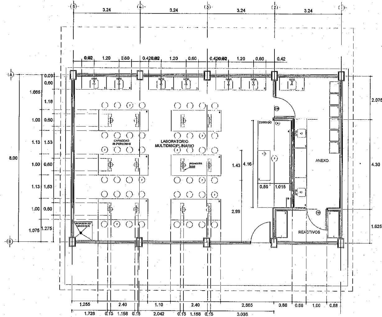
PLANTA ARQUITECTÓNICA LABORATORIO POLIFUNCIONAL
