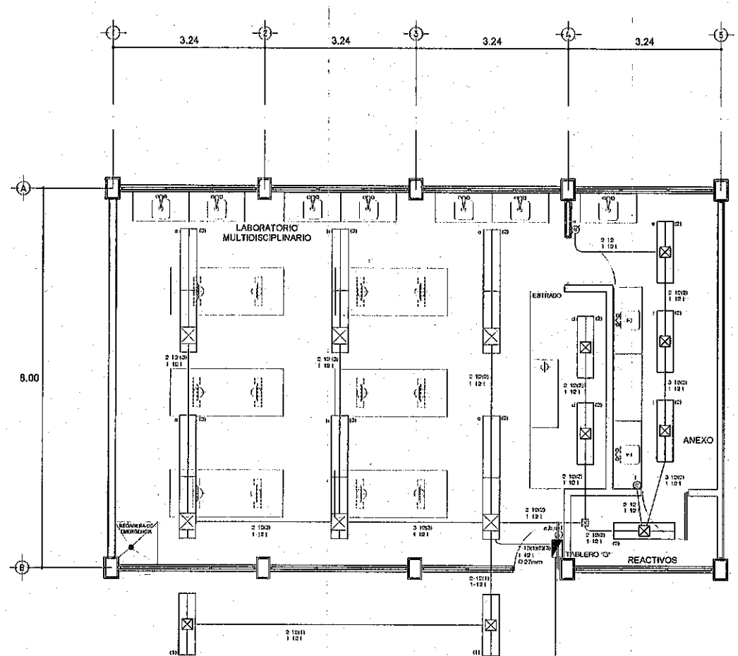
INSTALACIÓN ELÉCTRICA DE ALUMBRADO LABORATORIO POLIFUNCIONAL
