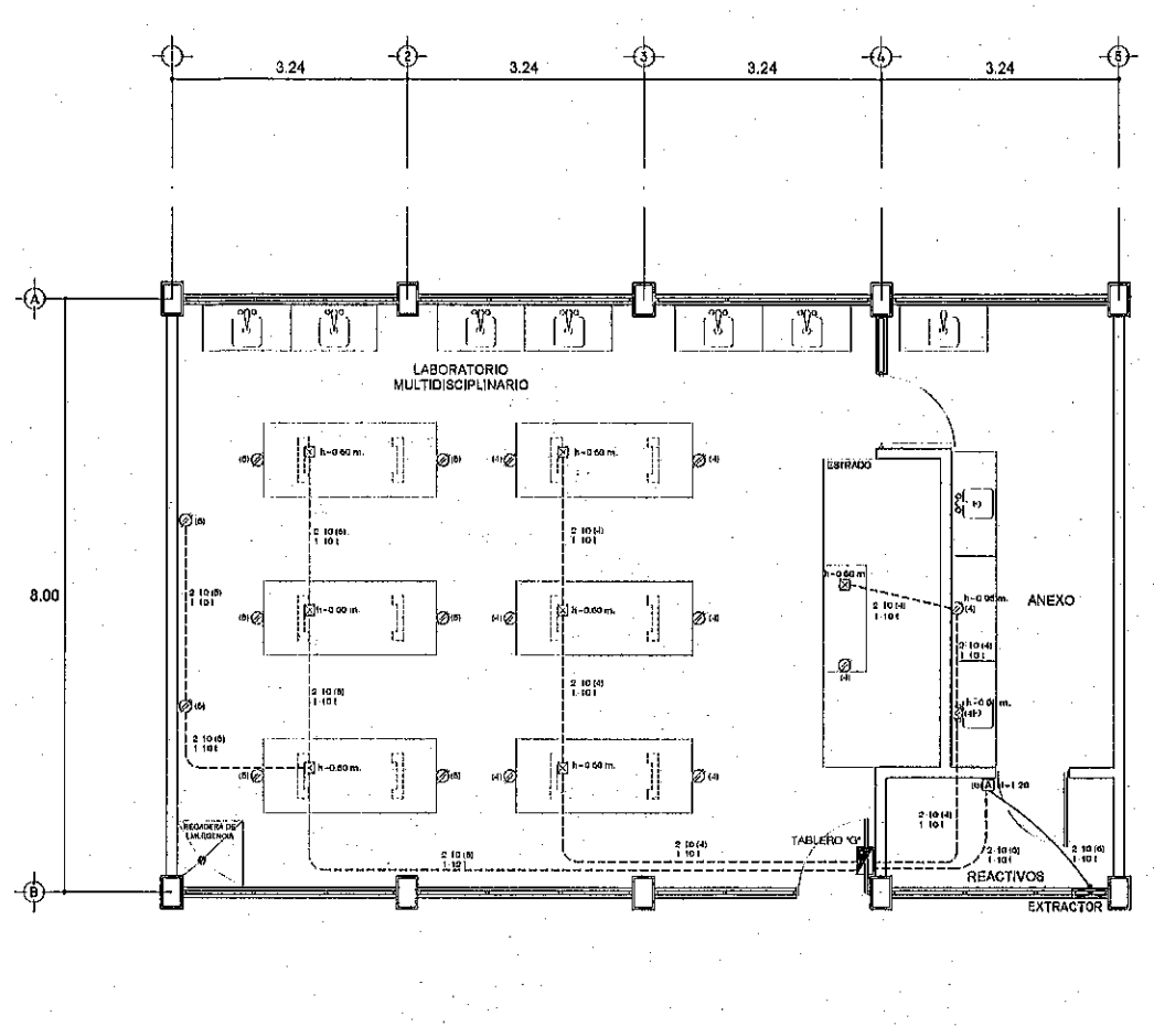
INSTALACIÓN ELÉCTRICA DE CONTACTOS LABORATORIO POLIFUNCIONAL
