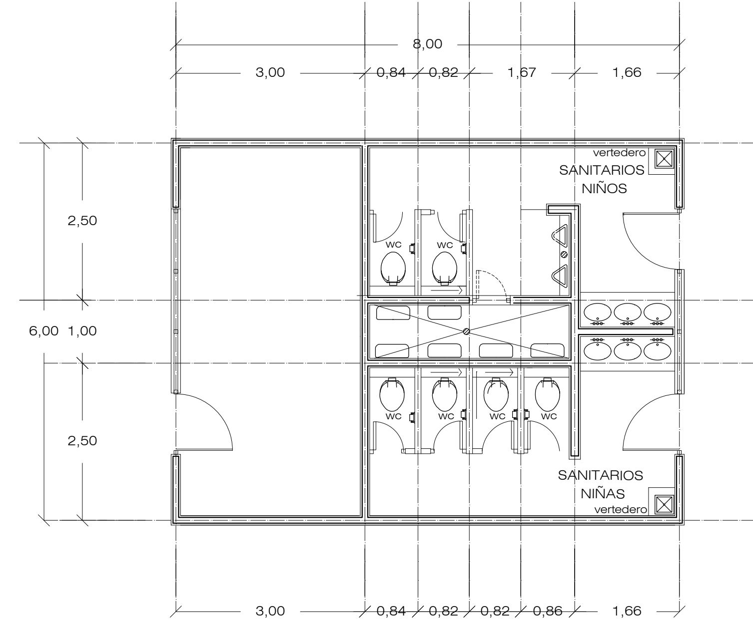
PLANTA ARQUITECTÓNICA REHABILITACIÓN SERVICIOS SANITARIOS
