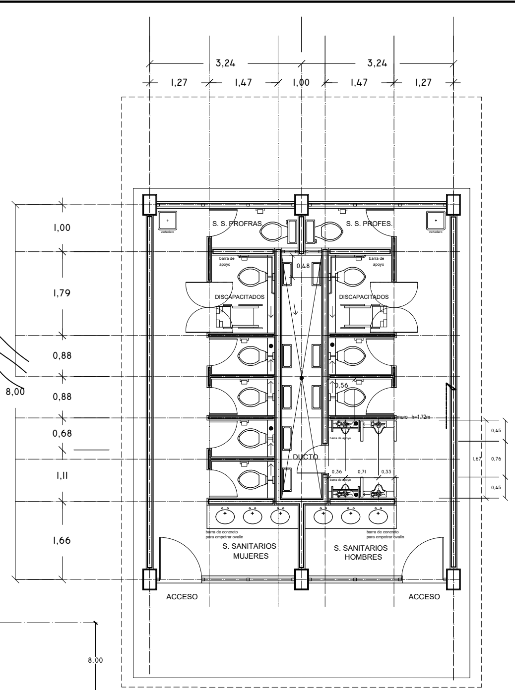
PLANTA ARQUITECTÓNICA REHABILITACIÓN SERVICIOS SANITARIOS
