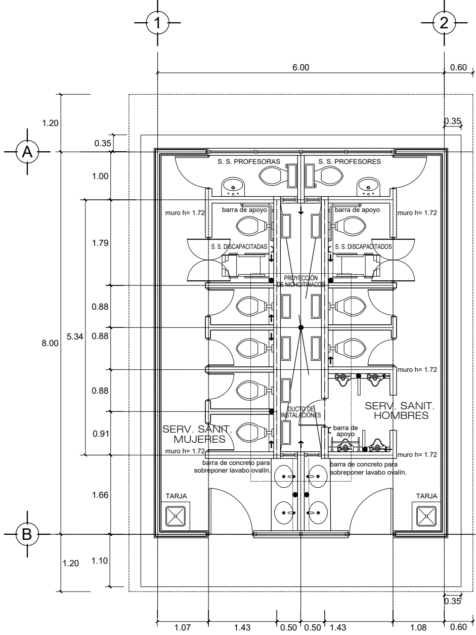
PLANTA ARQUITECTÓNICA REHABILITACIÓN SERVICIOS SANITARIOS
