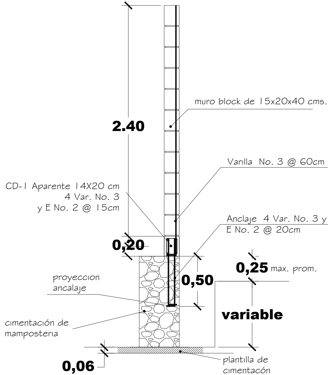
CORTE
