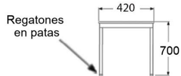
Vista lateral
