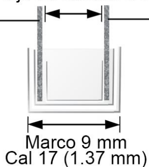
Corte
