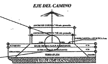
SECCIÓN TIPO BACHEO SUPERFICIAL
