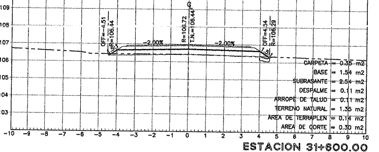
ESTACION 31+600.00
