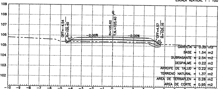
ESTACION 31+740.00
