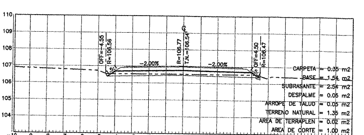
ESTACION 31+540.00
