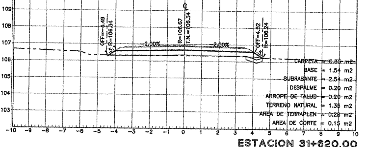
ESTACION 31+620.00
