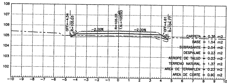
ESTACION 31+780.00
