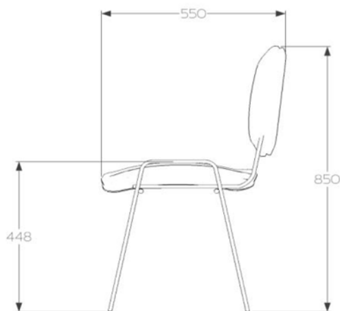
Vista Lateral
