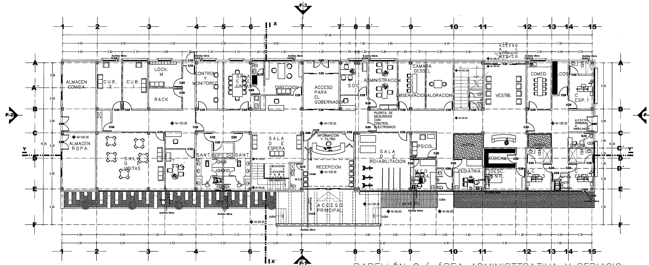
PABELLÓN C ( ÁREA ADMINISTTSATIVA Y SERVICIO MÉDICO). PLANTA BAJA
