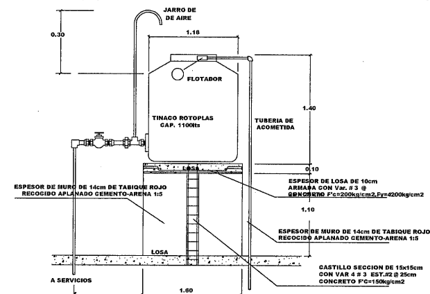
DETALLE DE TINACOS
