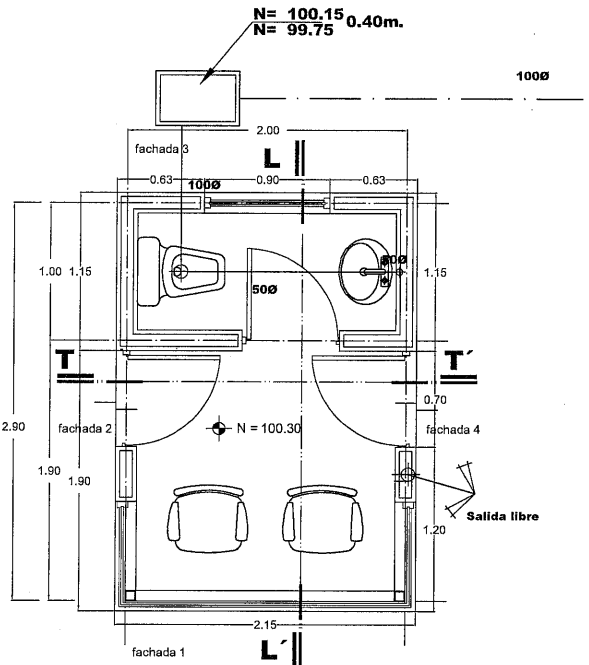
PLANTA BAJA SUP. CONSTRUIDA 6.56 M² ESCALA 1:25
