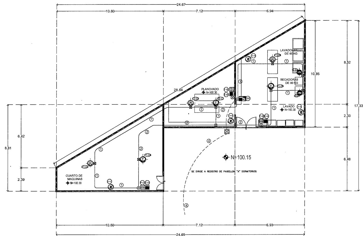
PLANTA BAJA
