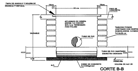
CORTE B-B
