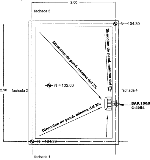
PLANTA DE AZOTEA ESCALA 1:25
