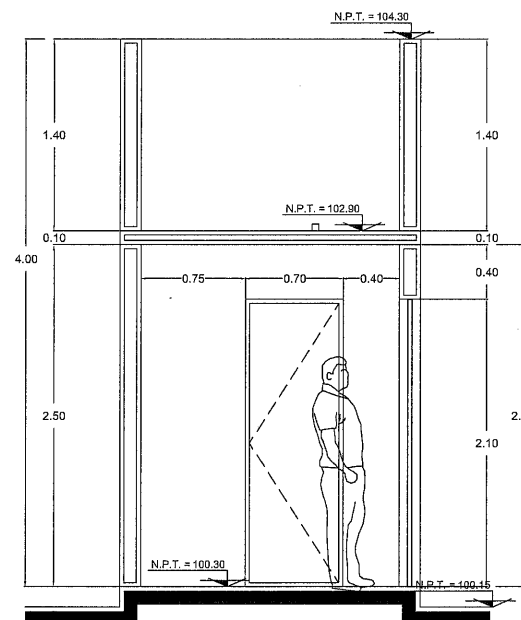
CORTE T-T' ESCALA 1:25
