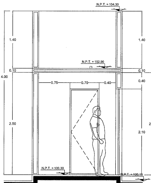
CORTE T-T' ESCALA 1:25
