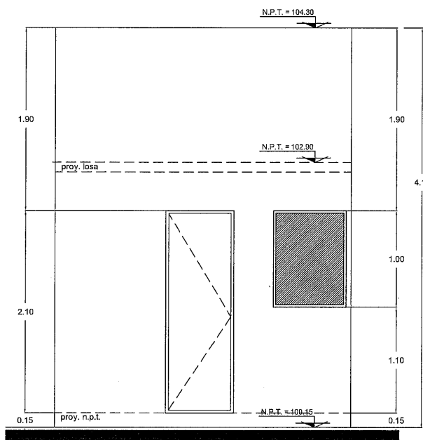
FACHADA 2 ESCALA 1:25
