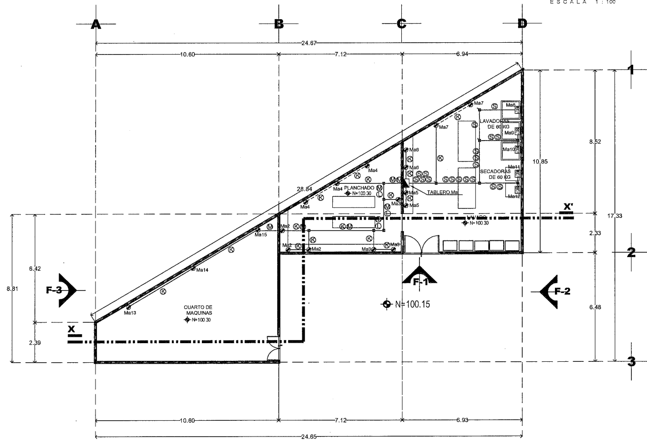
PLANTA BAJA
