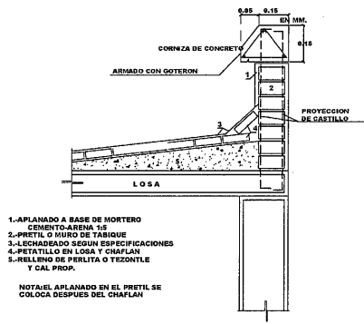
DET. CHAPLAN EN AZOTEA CON RELLENO Y PETATILLO CLAVE: DCHARP-01
