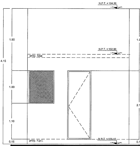
FACHADA 4 ESCALA 1:25
