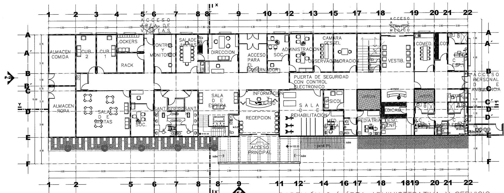
PABELLÓN C ( ÁREA ADMINISTTSATIVA Y SERVICIO MÉDICO). PLANTA BAJA SUPERFICIE CONST. 881.25M2 ESCALA 1:125
