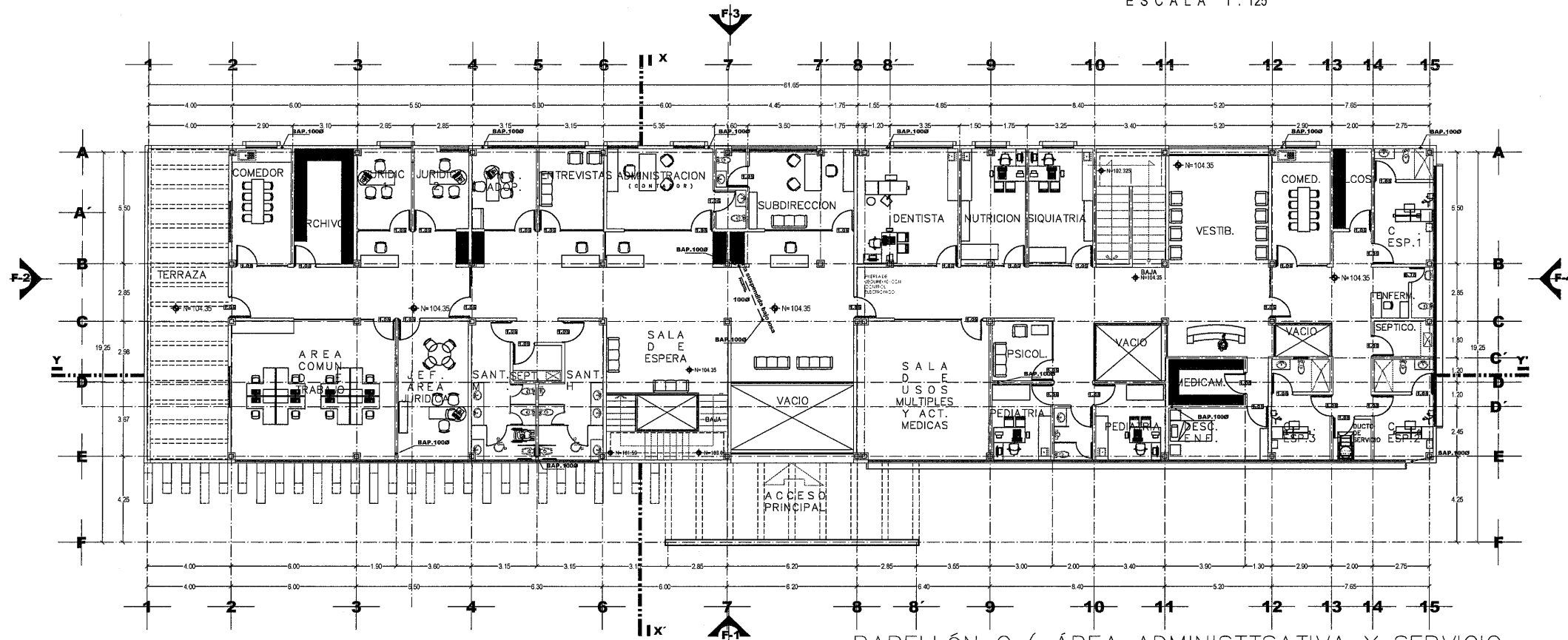
PABELLÓN C ( ÁREA ADMINISTTSATIVA Y SERVICIO MÉDICO). PLANTA ALTA
