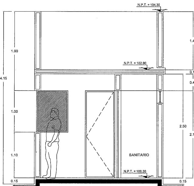
CORTE L-L' ESCALA 1:25
