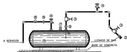
DETALLE DE TANQUE ESTACIONARIO
