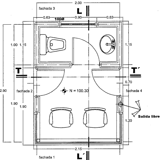
PLANTA BAJA SUP. CONSTRUIDA 6.56 M² ESCALA 1:25
