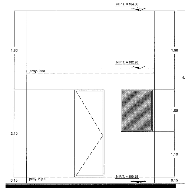
FACHADA 2 ESCALA 1:25
