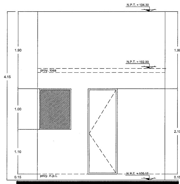
FACHADA 4 ESCALA 1:25
