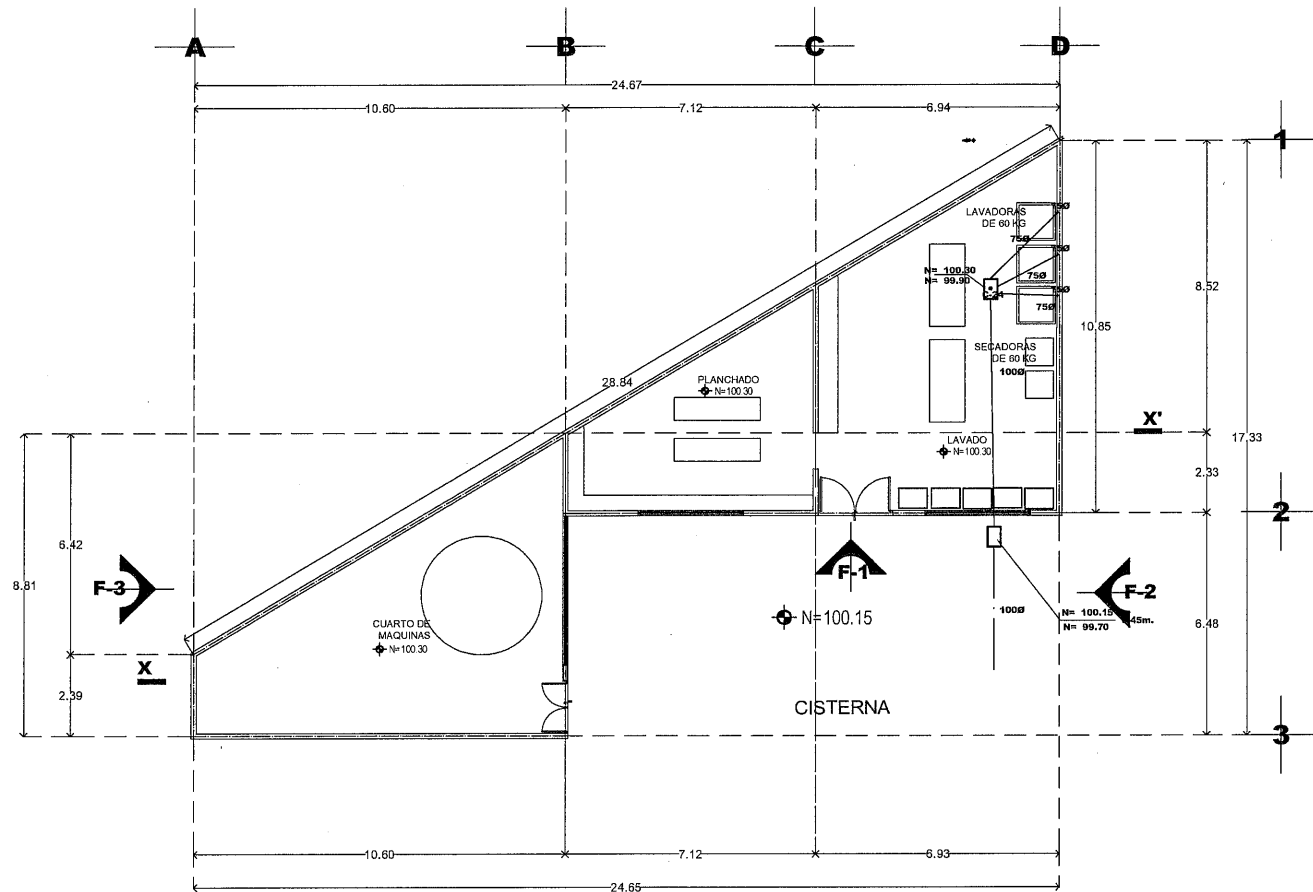
PLANTA BAJA
