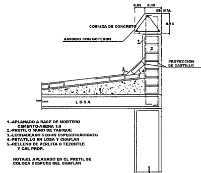
DET.CHAFLAN EN AZOTEA CON RELLENO Y PETATILLO CLAVE: DCHARP-01
