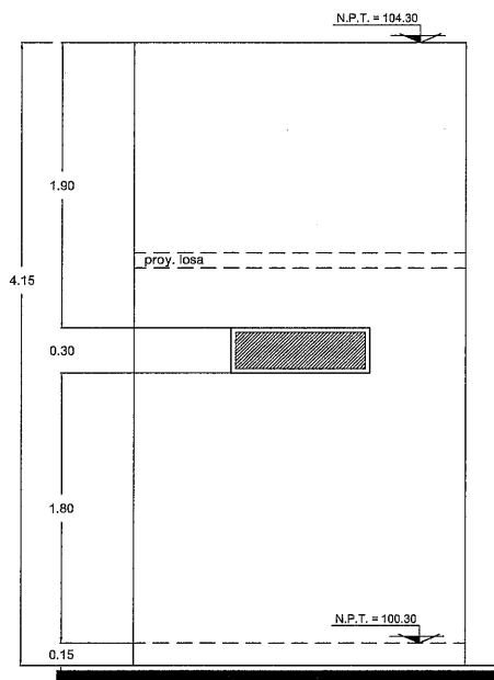
FACHADA 3 ESCALA 1:25
