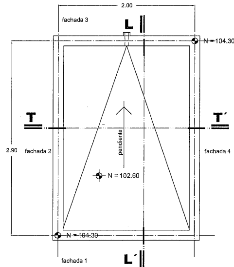
PLANTA DE AZOTEA ESCALA 1:25
