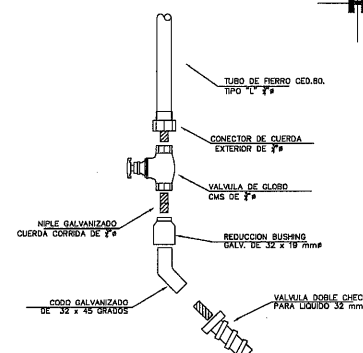
DETALLE DE ALIMENTACION (ACOMETIDA)
