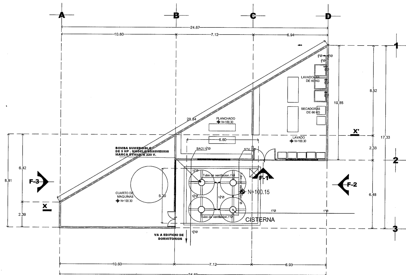
PLANTA BAJA
