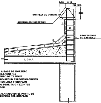
DET. CHAPLAN EN AZOTEA CON RELLENO Y PETATILLO CLAVE: DCHARP-01
