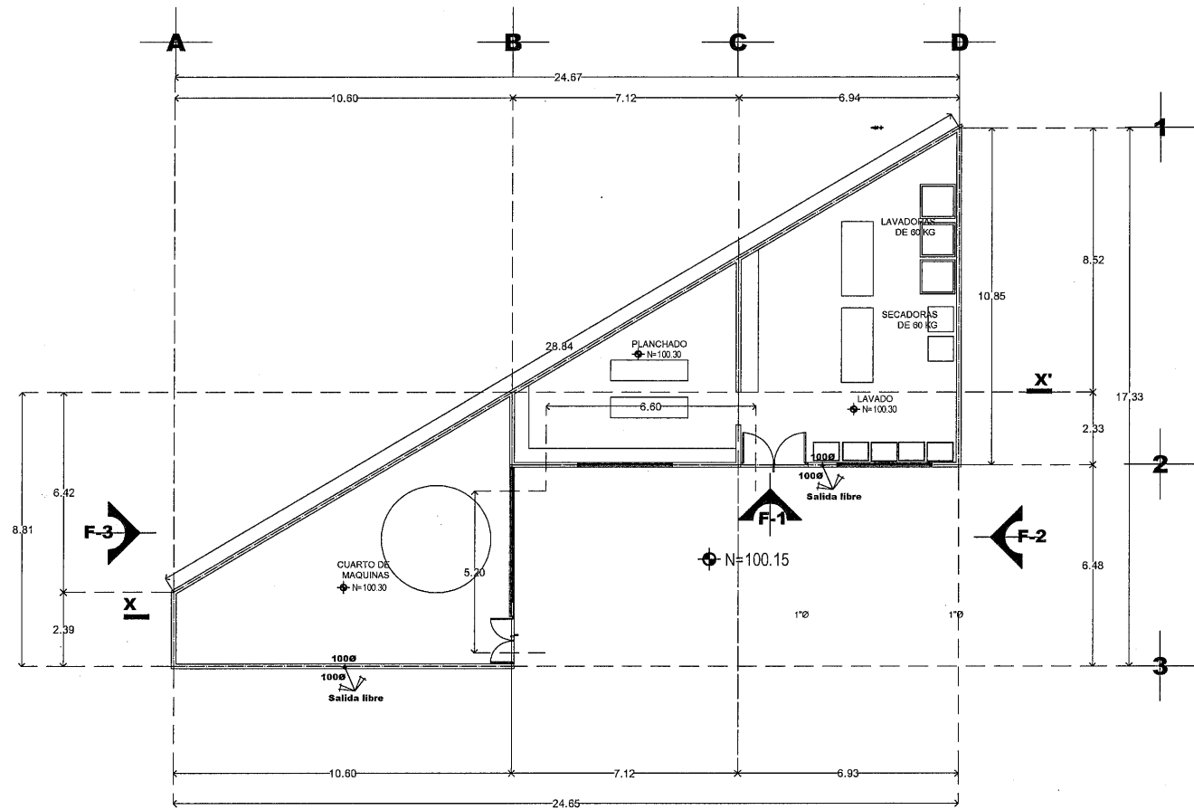
PLANTA BAJA
