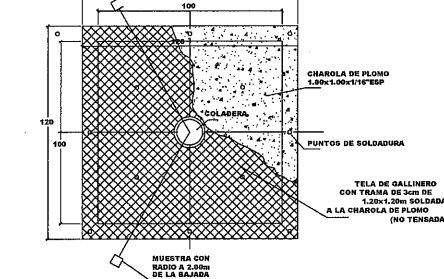
DETALLE DE BAP. PARA CENTRO EN AZOTEA CON COLADERA HELVEX MOD C-444 CLAVE: DBPCA-01
