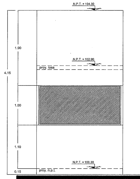
FACHADA 1 ESCALA 1:25
