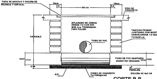
CORTE B-B
