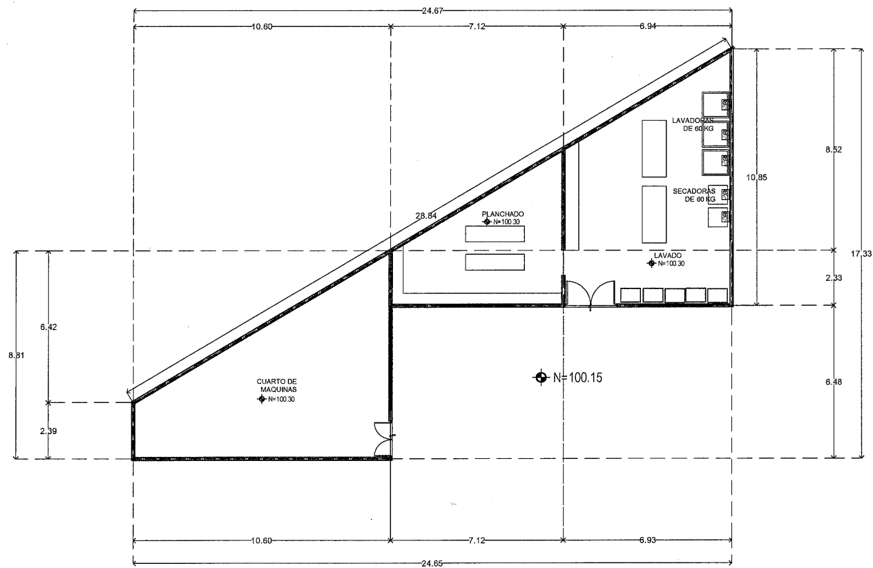
PLANTA BAJA SUPERFICIE CONST. 157.46M2 ESCALA 1:100
