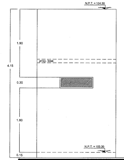
FACHADA 3 ESCALA 1:25
