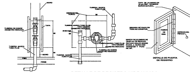
DETALLE DE REGISTRO HIDRAULICO
