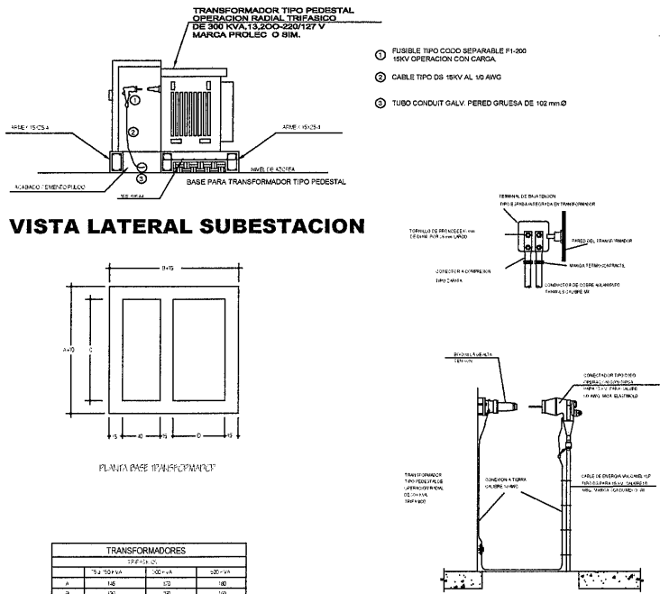
DETALLE SUBESTACION ELECTRICA TIPO PEDESTAL
