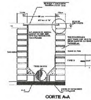
CORTE A-A
