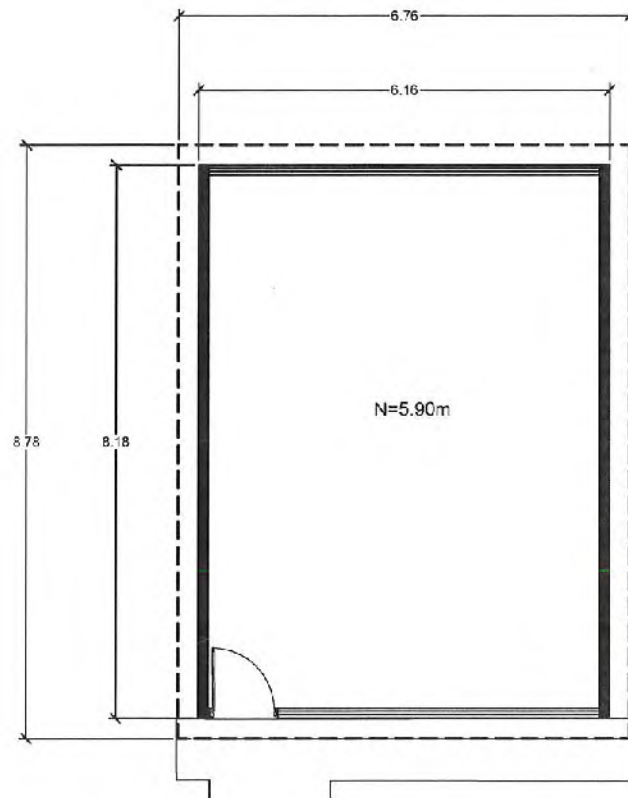
PLANTA ALMACEN SUPERFICIE A REMODELAR: 50 M2 1/30
