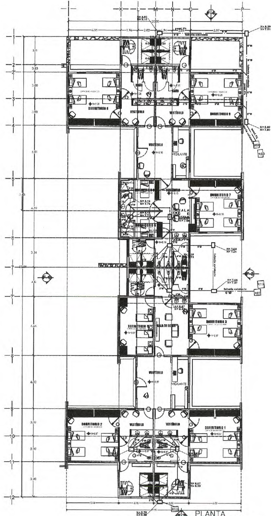
PLANTA MODULO "F" ARQUITECTÓNICA
