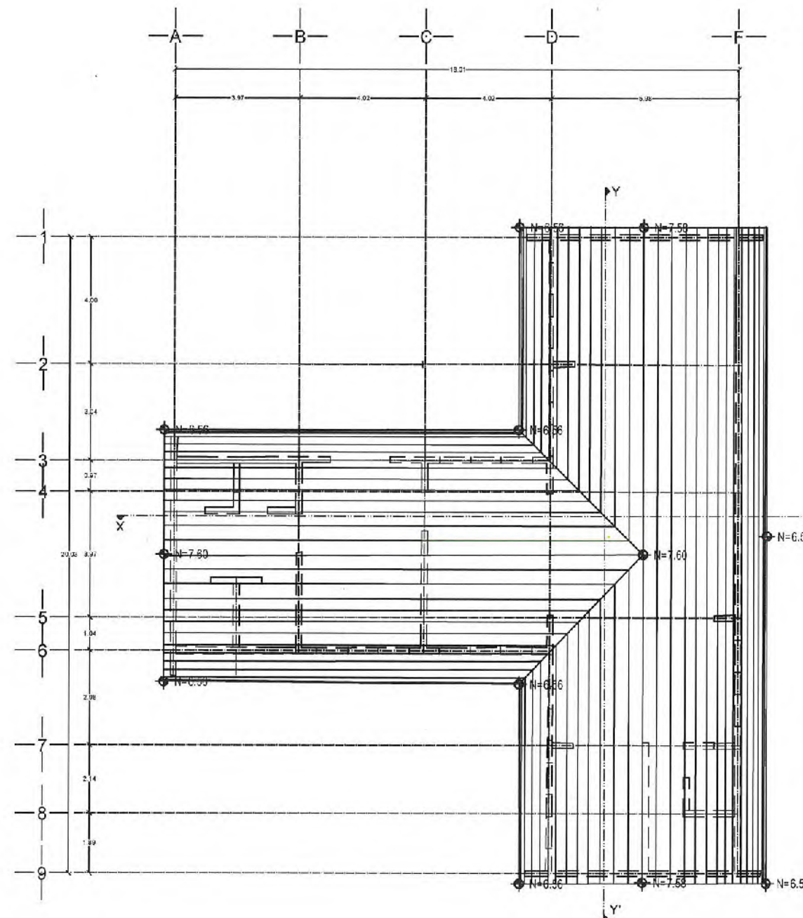
PLANTA AZOTEA DE MODULO "A" DIRECCIÓN SUPERFICIE A REMODELAR: 213.73 M2
