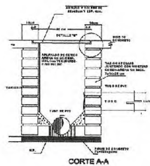
CORTE A-A
