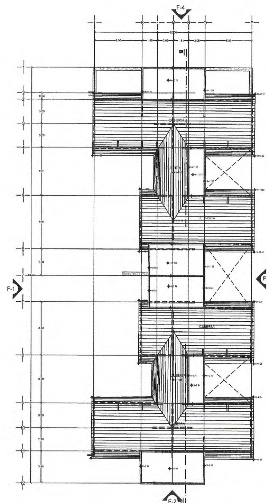
PLANTA DE AZOTEA DE MÓDULO "F" DORMITORIOS SUPERFICIE PROYECTADA = M 2
