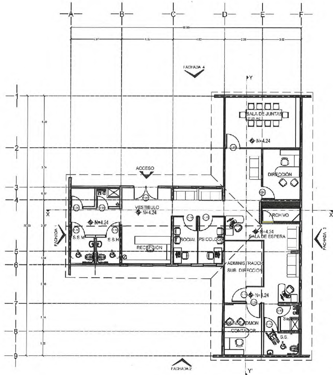
PLANTA ARQUITECTÓNICA DE MODULO "A" DIRECCIÓN SUPERFICIE A REMODELAR: 293.73 M2
