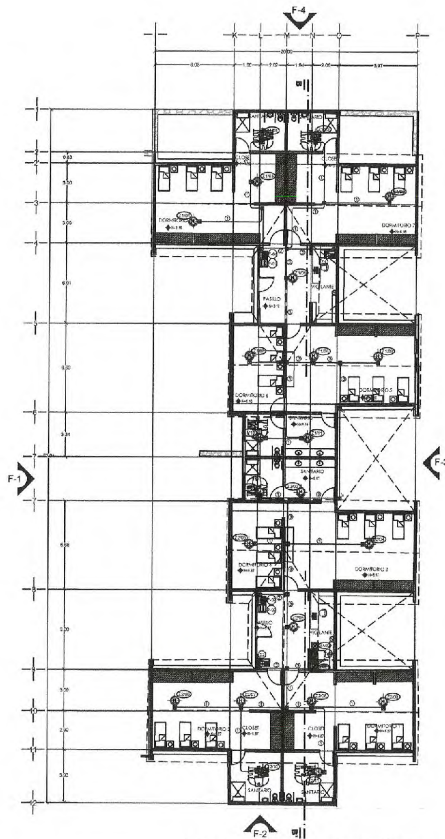
PLANTA ARQUITECTÓNICA DE MÓDULO "F" DORMITORIOS SUPERFICIE PROYECTADA - M2 1.928
