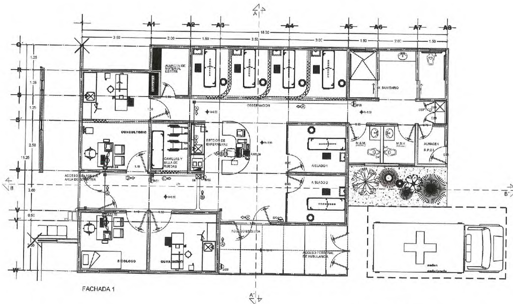
PLANTA ARQUITECTONICA
