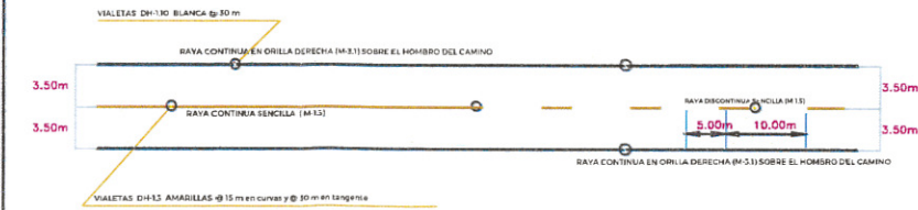
DETALLE DE SEÑALAMIENTO HORIZONTAL
