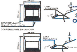
DETALLE DE BOTONES REFLEJANTES (DH-1)
